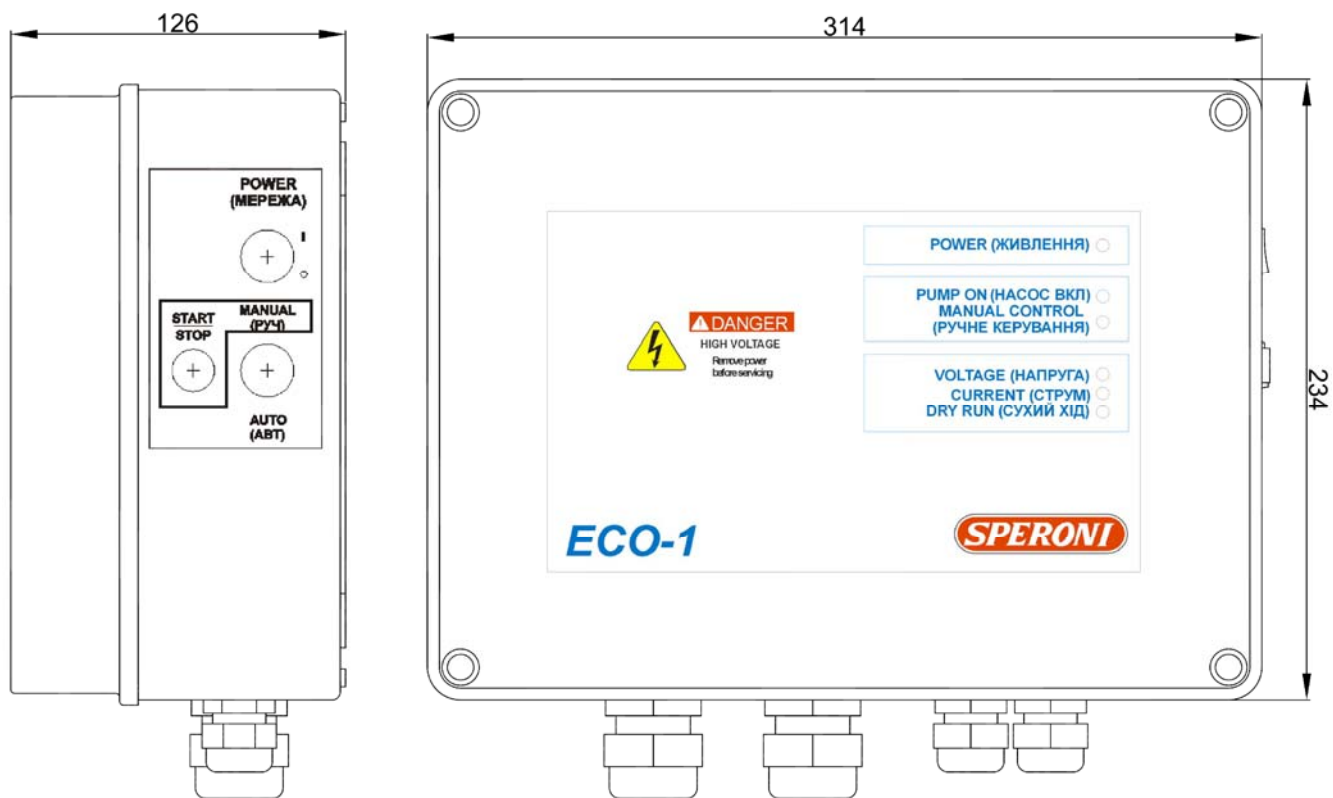
Рис. 1 Устройство ECO-1
